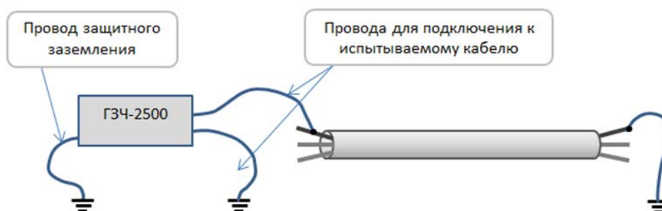
Рисунок 3. Трассировка кабеля.
